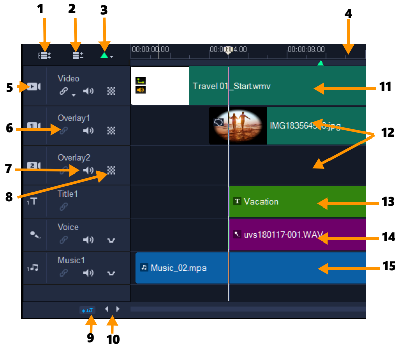
Tijdlijnweergave van Corel VideoStudio
